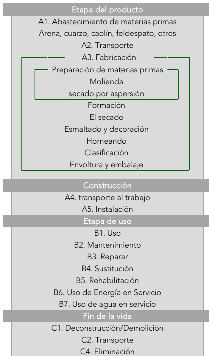
Figura 1. Diagrama con los límites del sistema, pasos y procesos para la producción de 1 m 2 de baldosa cerámica B1a (20 mm)
