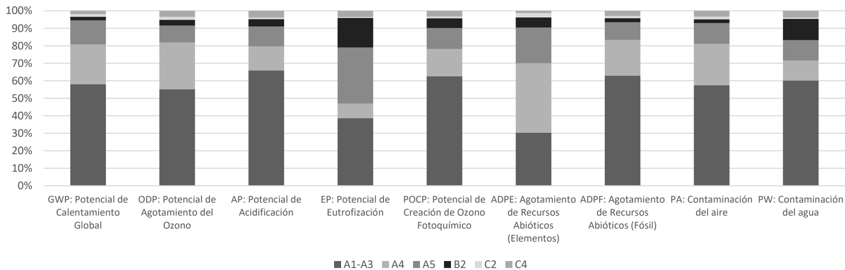
Figura 4. Contribución relativa de los módulos de Ciclo de Vida a los impactos ambientales potenciales de 1 m 2 de baldosas cerámicas Newker Bla (20 mm) con destino España.
