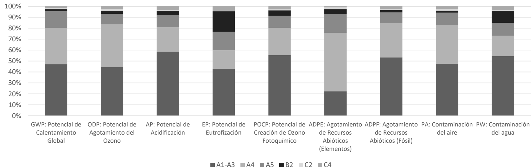
Figura 3. Contribución relativa de los módulos de Ciclo de Vida a los impactos ambientales potenciales de 1 m 2 de baldosas cerámicas Newker Bla (20 mm) con destino Francia.
