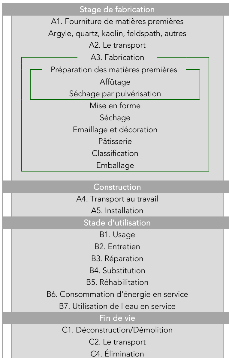
Figure 1. Schéma avec les limites du système, les étapes et les processus pour la production de 1 m 2 de carreaux de céramique Bla (20 mm)
