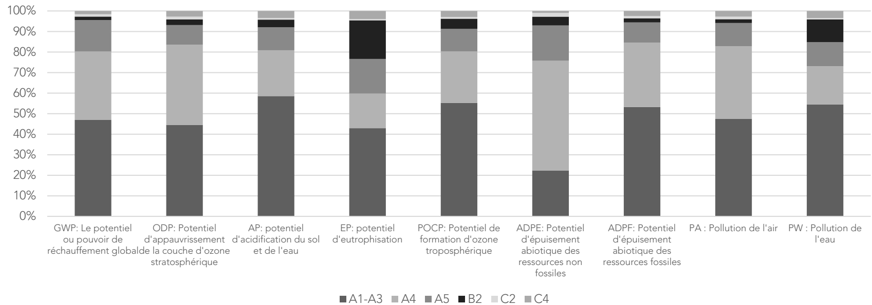
Figure 3. Contribution relative des modules du cycle de vie aux impacts environnementaux potentiels de 1 m 2 de dalles céramiques Newker Bla (20 mm) avec destination France.
