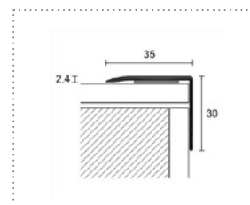
PERFIL DE PELDAÑO METÁLICO AUTOADHESIVO* SELF-ADHESIVE STEP PROFILE* L: 270cm.
