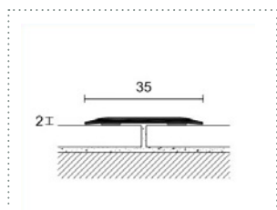
PERFIL DE TRANSICIÓN AUTOADHESIVO* SELF-ADHESIVE TRANSITION PROFILE* L: 270cm.
